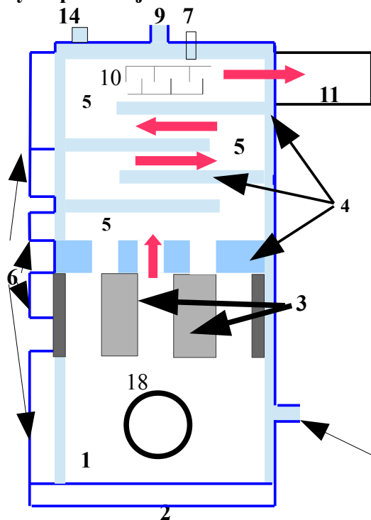
rys.1 przekrój kotła
